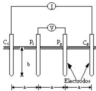
Fig. 4. Wenner configuration
