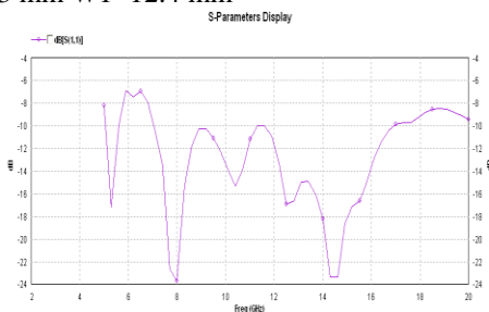
Fig. 4.1.2 Iteration 1 S-Parameters
